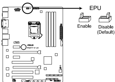
P8Z77-V LE EPU switch
